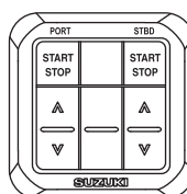
デュアルエンジン用
